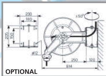
Optional version with lateral protective covers and anti-derailment bracket Versione optional con carter laterali di protezione e staffa antiscurrimento
